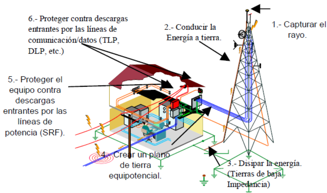
Figura 1 - Modelo de Protección eléctrica en instalaciones de sistemas de cómputo y comunicaciones
