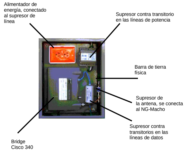
Figura 8 - Estándar de conexión en caja NEMA de los enlaces inalámbricos de la RIUADY
