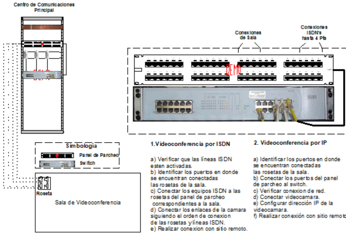
Figura 9 - Estándar de conexiones para videoconferencia
