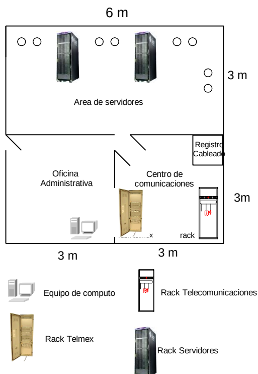
Figura 6.- Estándar para un centro de comunicaciones en DES
