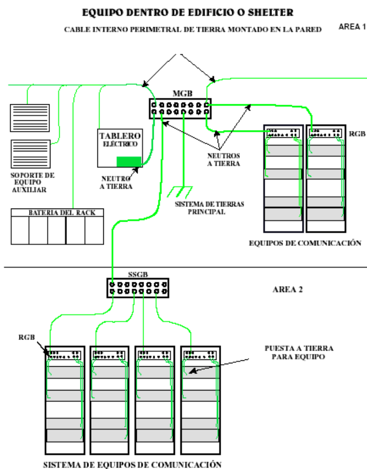
Figura 2 - Sistemas de tierra en centro de comunicaciones
