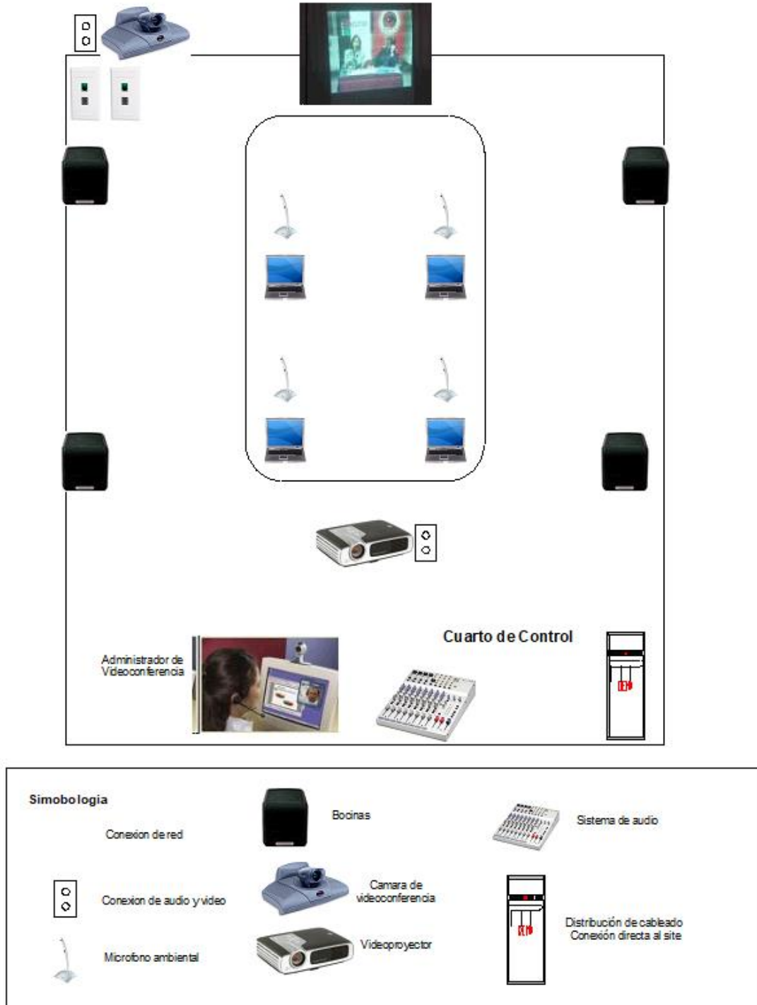
Estándar de Sala Videoconferencia de la RIUADY
