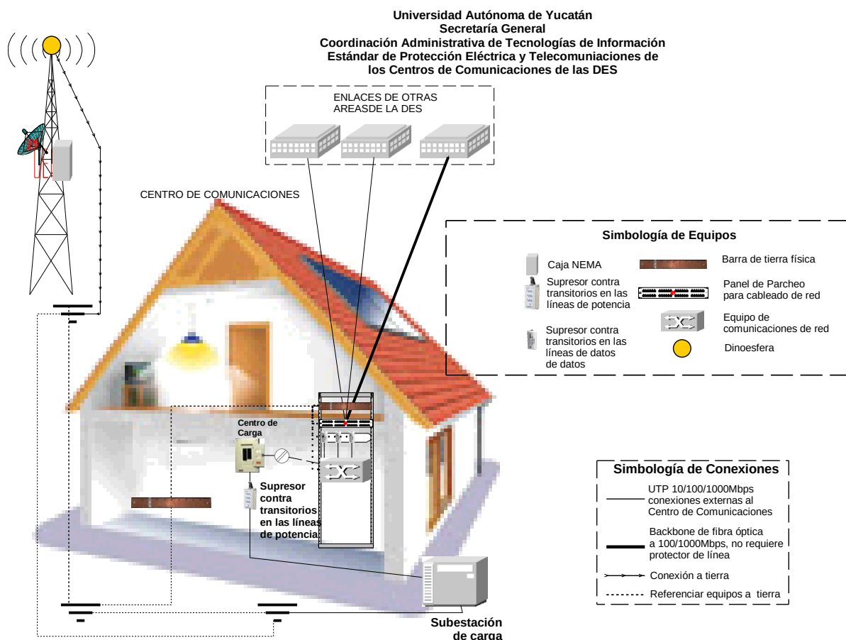
Figura 7 - Estándar de protección eléctrica y telecomunicaciones de los centros de telecomunicaciones de las DES
