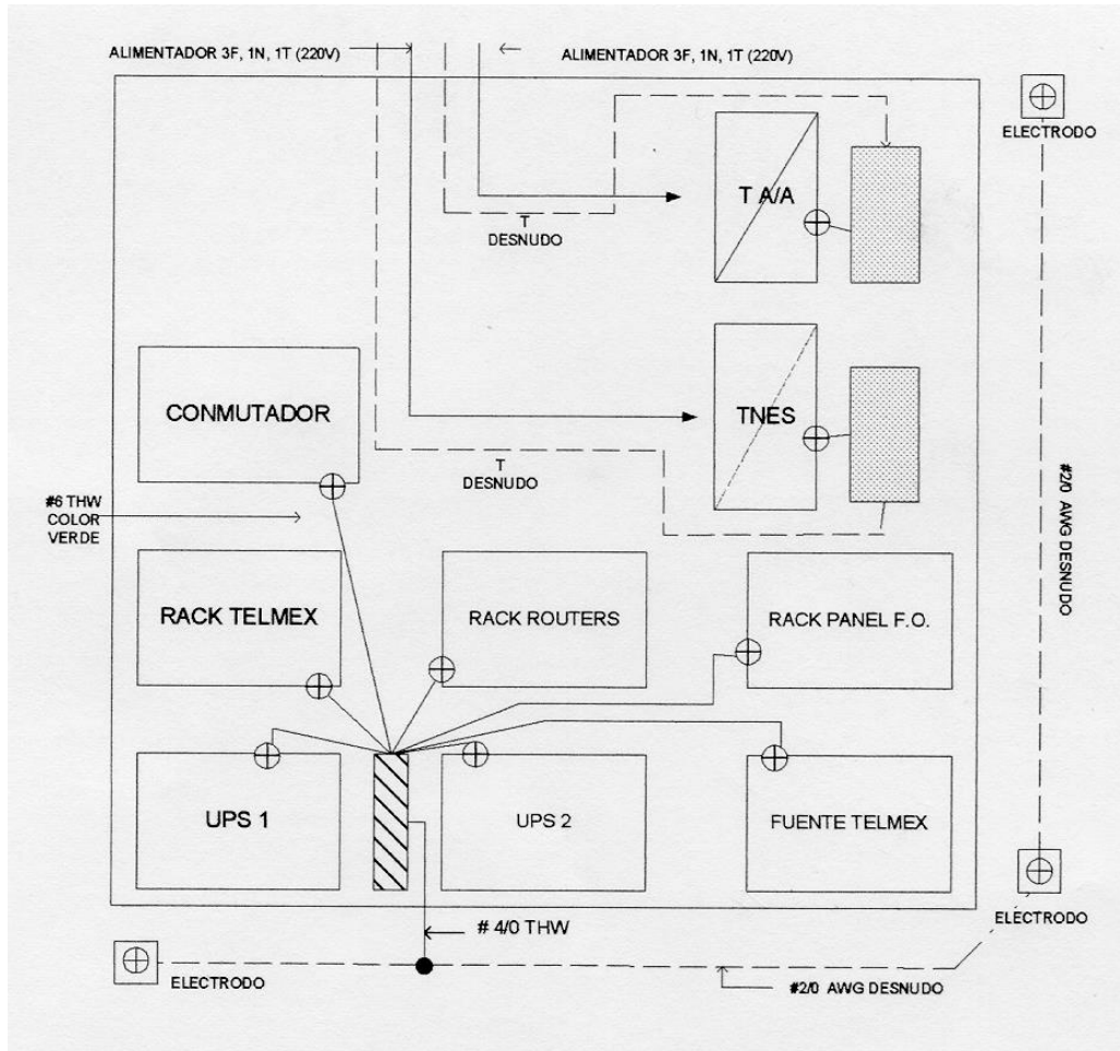
Figura 3 - Sistemas de tierra en centro de comunicaciones, planos
